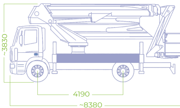
IVECO EUROCARGO
